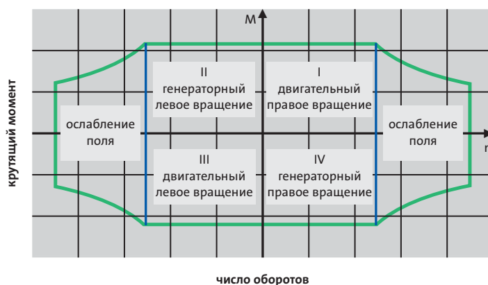
Области применения приводов с регулируемым числом оборотов
